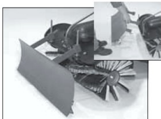
2. Установите нож отвала на стержни.
